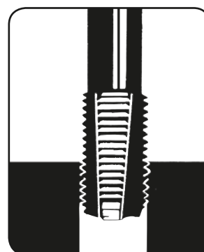
2. Gjenge opp hullet med den medfølgende spesialtappen.
